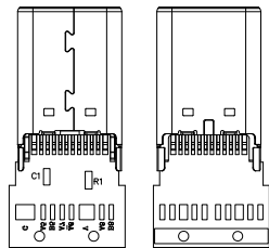
Conn.1_USB TYPE-C (MALE)
